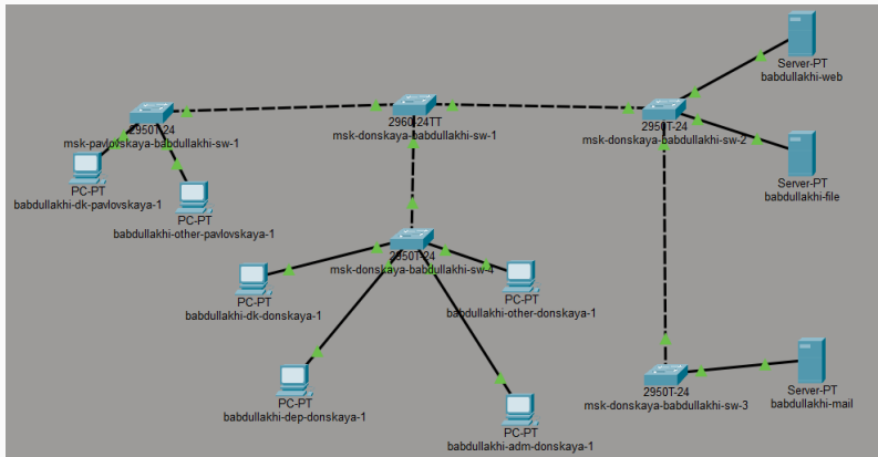
Рис. 1: Топология сети L1
